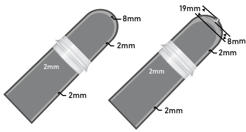
HIGH RING: L'anello è collocato a 18 cm dal centro dell'estremità distale.
